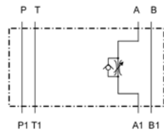
Schaltbild RD
